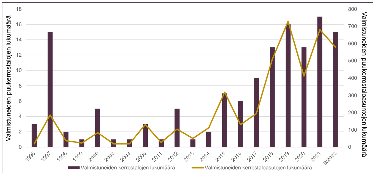
Kuva 2. Valmistuneiden puukerrostalojen ja puukerrostaloasuntojen lukumäärä 1996-9/2022. 8
