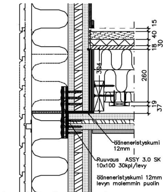
Kuva 11. Julkisivun sauma
