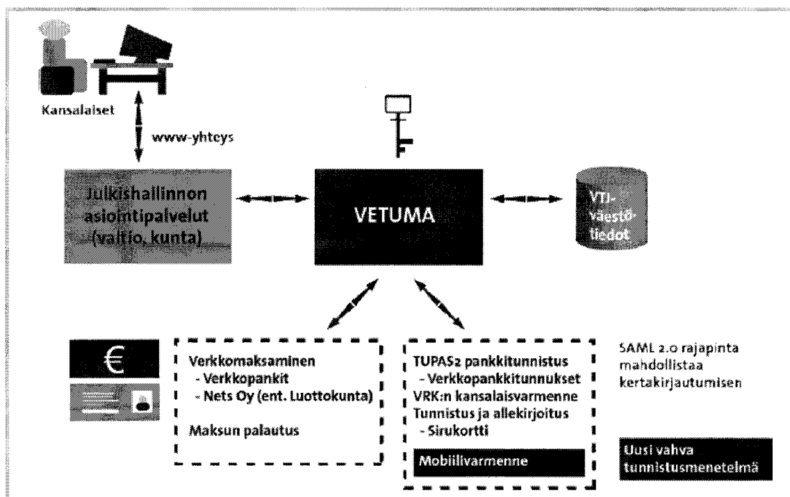
Kuva 1b Vetuma-palvelun toimintaperiaate
