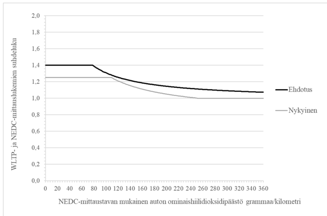
Kuva 1. WLTP- ja NEDC-mittaustapojen mukaisten hiilidioksidipäästöjen suhde eri päästötasoilla nykyisessä ja ehdotetussa sopeutuksessa.
