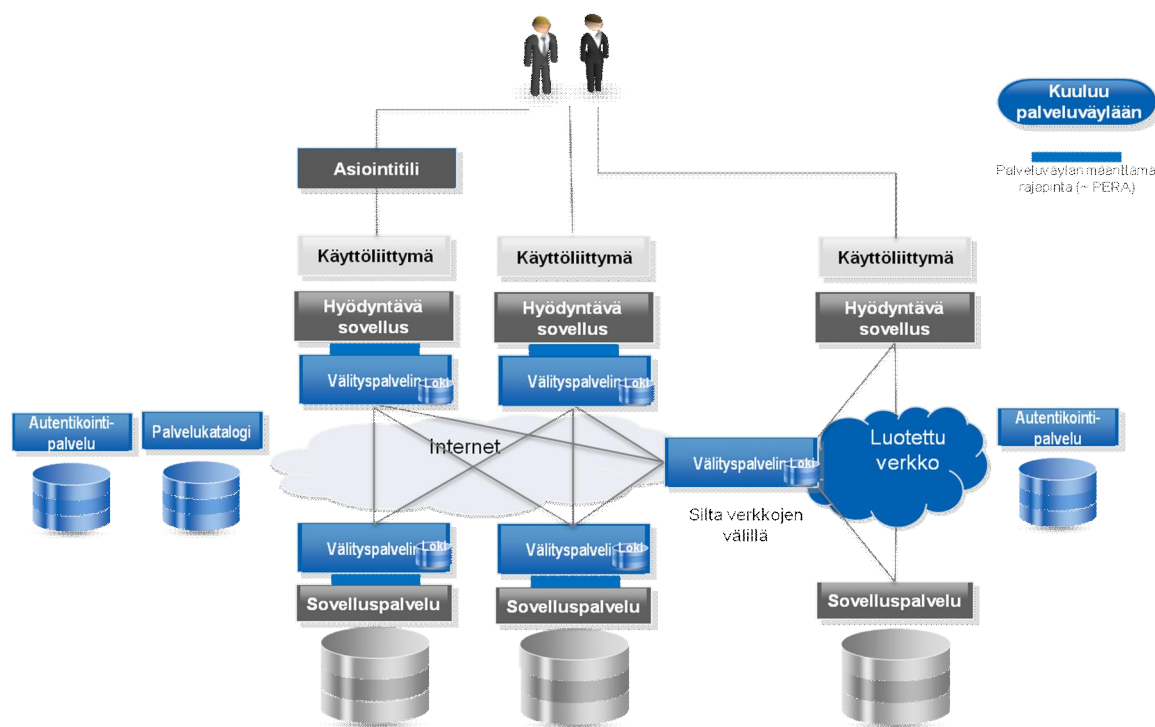
Kuva 6: Palveluväylän viitearkkitehtuuri, jatkotyöstöön valittu skenaario
