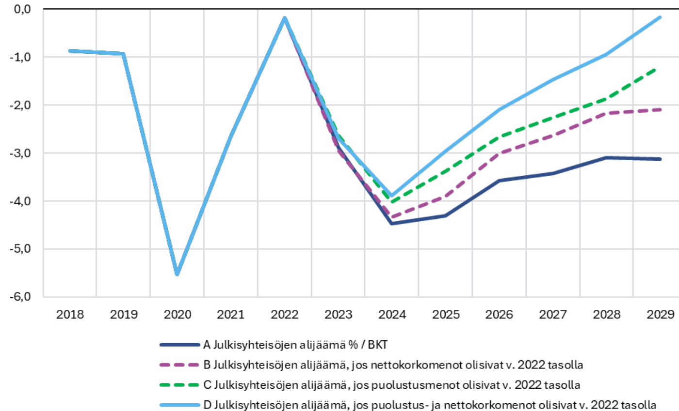
Julkisyhteisöjen alijäämä, % suhteessa BKT:hen
