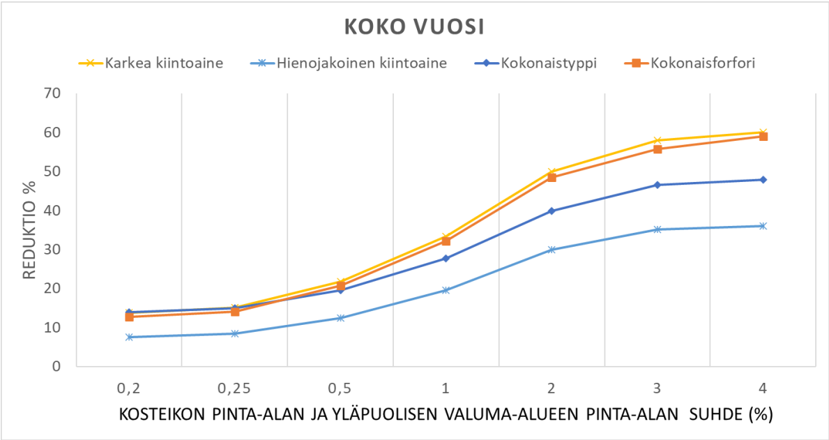
Kuva 6. Kosteikon pinta-alan ja yläpuolisen valuma-alueen pinta-alan suhteen merkitys kosteikon kykyyn pidättää kiintoaineita ja ravinteita.
